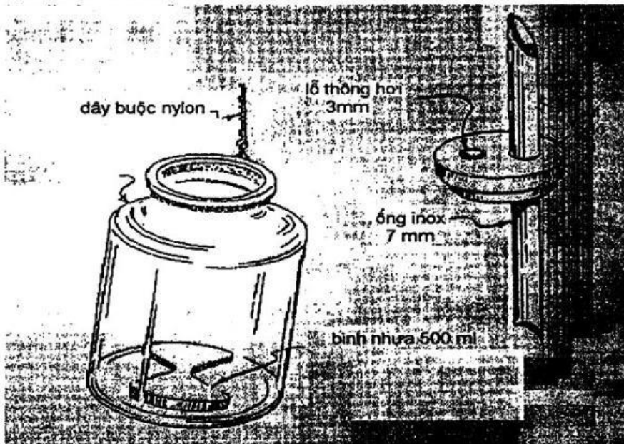
Hình A.2 - Chai lấy mẫu phân bón lỏng
