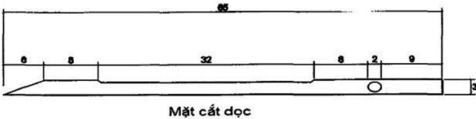
Hình A.7 - Xiên lấy mẫu 1 điểm (bao 10kg)
