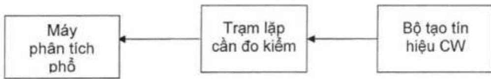
Hình D.5 - Sơ đồ đo xuyên điều chế đầu vào
